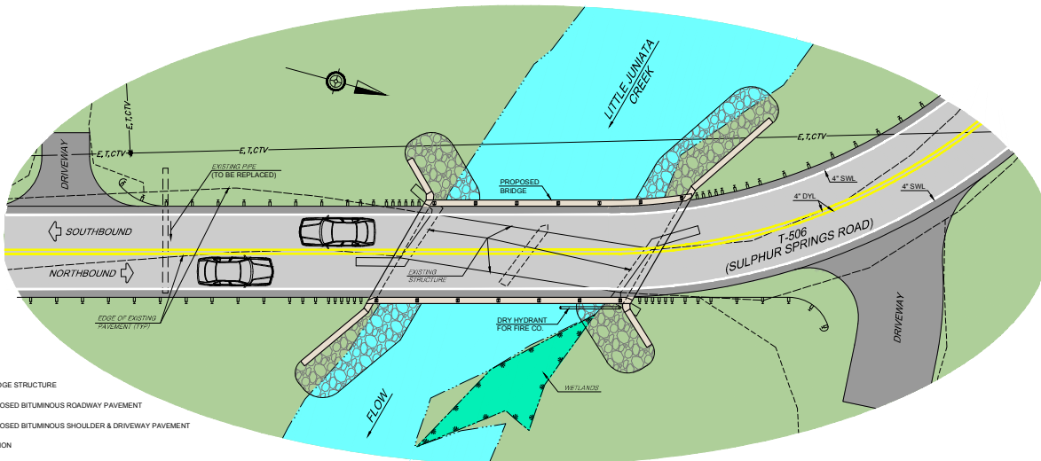
PLAN SCALE: 1" = 10'
